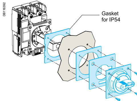
EZC250/EZCV250.
