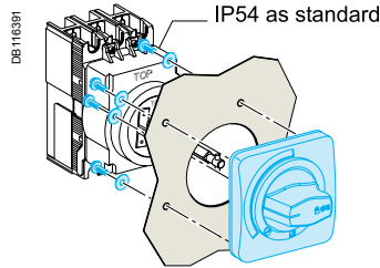
EZC100.
