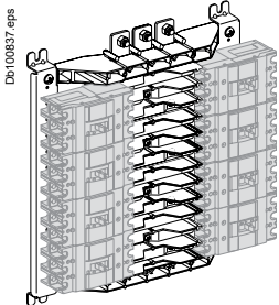
8 ways (3P)
